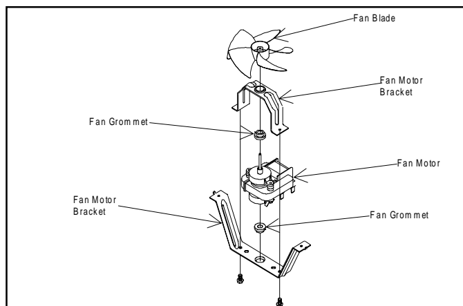
Evaporator Fan
