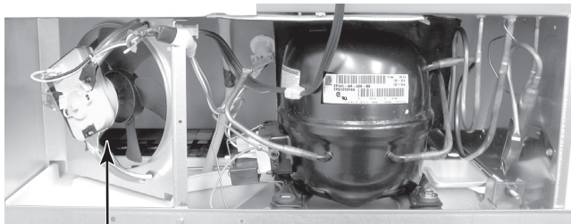
Condenser Fan Motor
